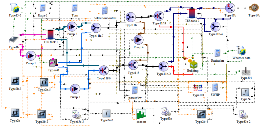
b) Parallel IX-SAASHP
