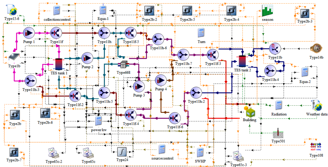
a) Serial IX-SAASHP
